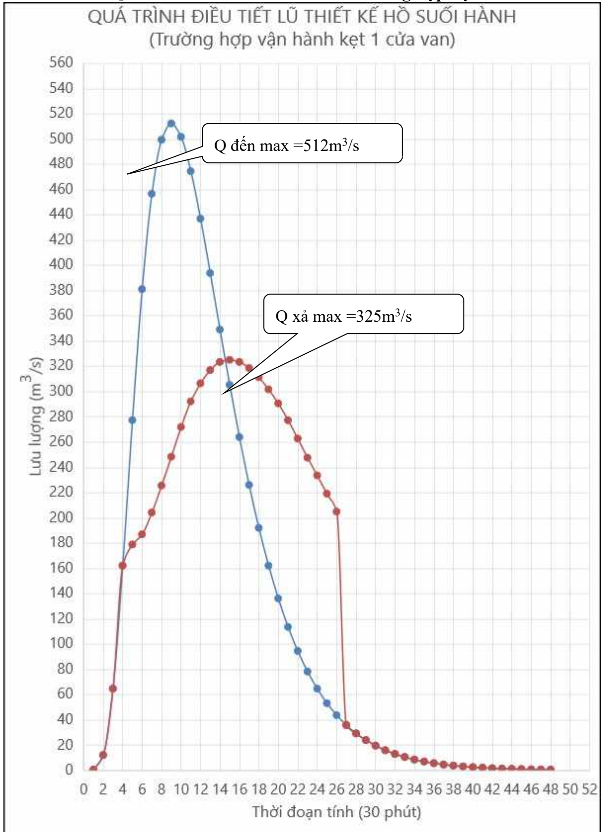
Hình PL 4.2: Quá trình điều tiết lũ thiết kế - trường hợp kẹt 1 cửa van
